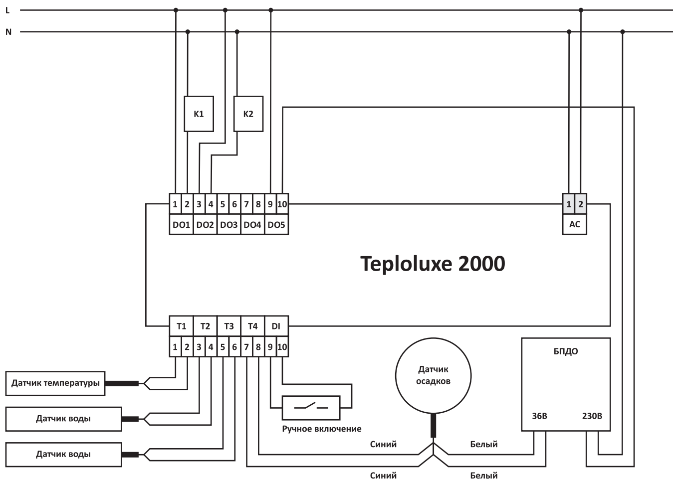
Рис. 3.1.1. Принципиальная схема подключения в режиме «Кровля»
